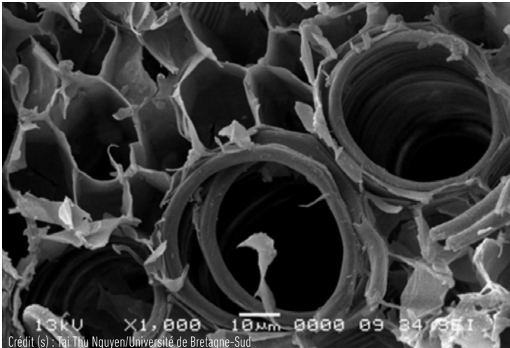
← Ces deux images obtenues en microscopie électronique à balayage montrent la microstructure d'une tige de chanvre vue en coupe.
